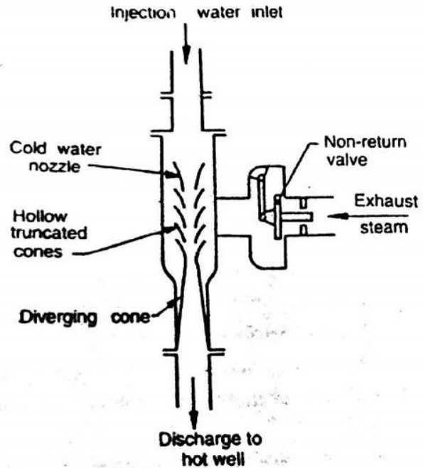
Fig. 6.4 Ejector Condensers
